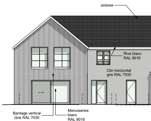
Façade Sud Ouest
