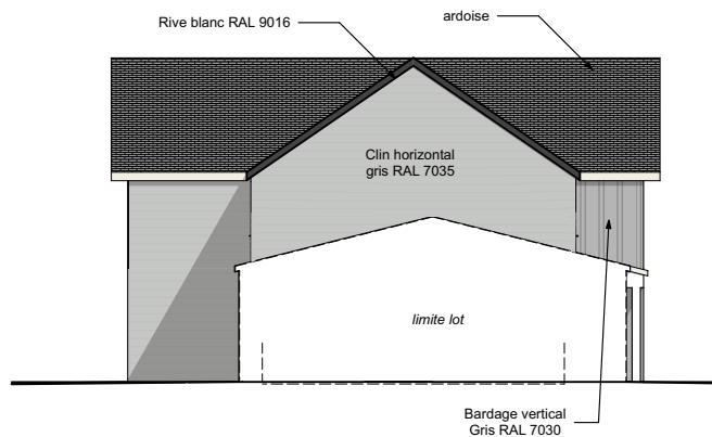
Façade Sud Est
