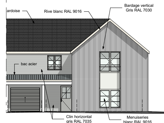
Façade Nord Est
