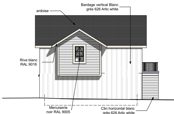
Façade Sud Ouest
