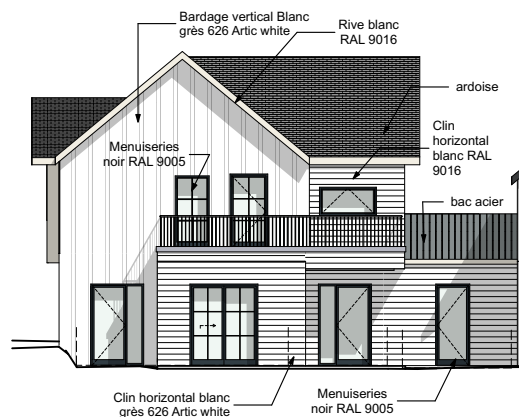
Façade Sud Est
