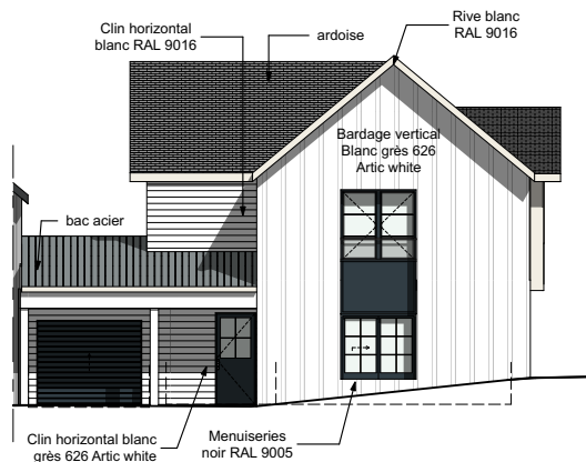
Façade Nord Ouest
