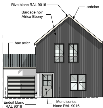
Façade Nord Est
