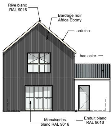
Façade Sud Ouest
