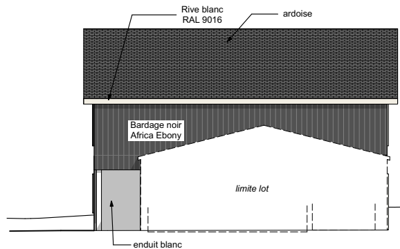
Façade Nord Est
