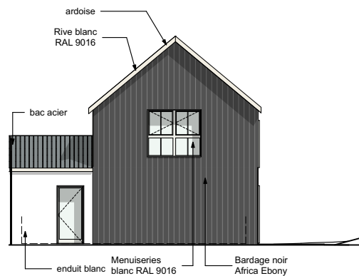
Façade Nord Ouest
