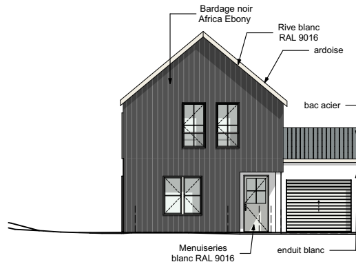
Façade Sud Est
