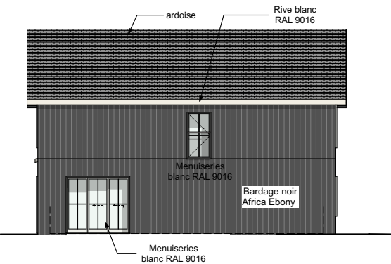
Façade Sud Ouest
